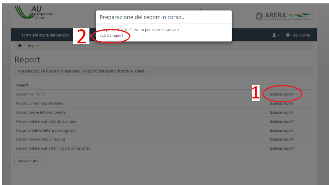
Fig. 15 Sezione report
